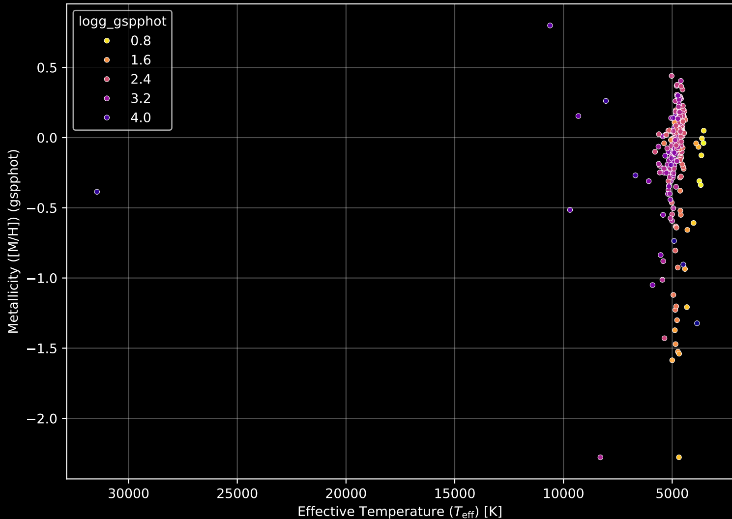
APOGEE DR17 Field: [005-08] Stellar Population Parameters (n= 274)
